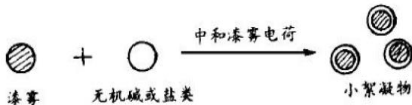
图3-4 高效喷漆废气吸收塔中漆雾被吸收示意图
