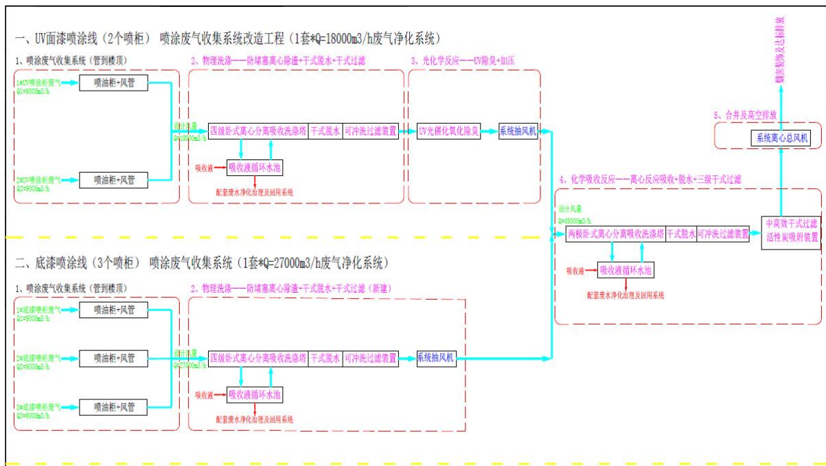
图3-3 喷涂烘干废气治理设施工艺流程图
